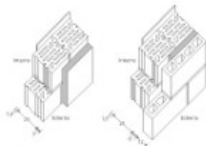
Facciata frontale con elementi 4x2,5 m con isolamento a cappotto
